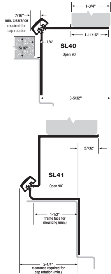
Fig. 2 Door Open 90°
