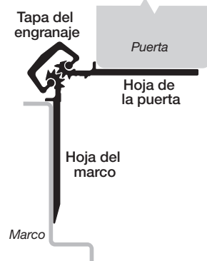
Fig. 2 Puerta abierta a 90°
