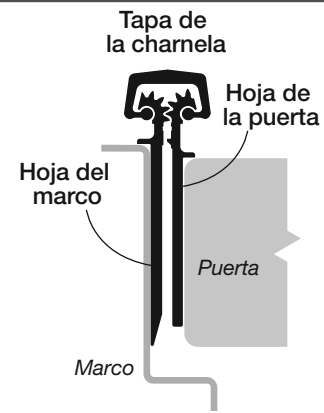
Fig. 1 Posición de puerta cerrada
