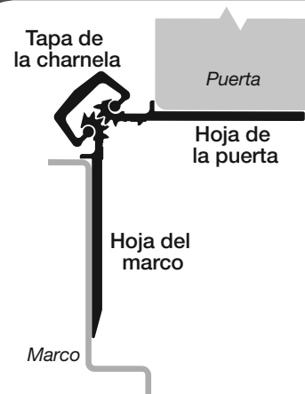
Fig. 2 Puerta abierta a 90°
