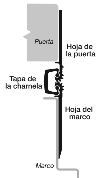
Fig. 3 Puerta abierta a 180°
